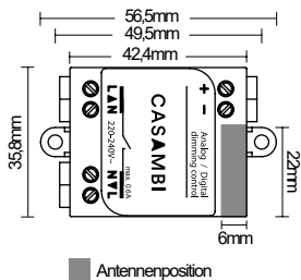
Antennenposition
